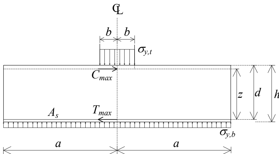
Figur 3 Ækvivalent kraftpar
