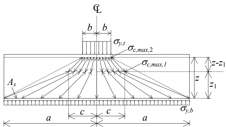
Figur 7 Vifteformet spændingsfordeling. To vifter
