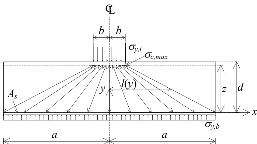
Figur 4 Vifteformet spændingsfordeling. En vifte
