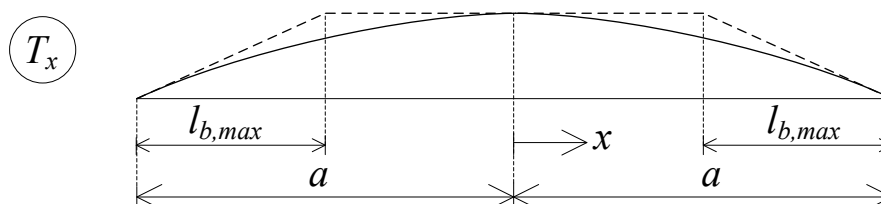
Figur 6 Fuldt optrukken linje: Variation af trækraft i værarmering. Stiplet linje: Kapacitet af tværarmering
